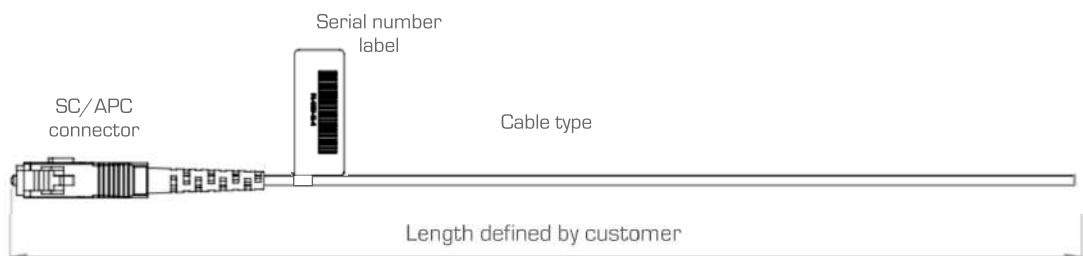
Fig. 1 3.0mm & 4.8mm MDU CABLE
